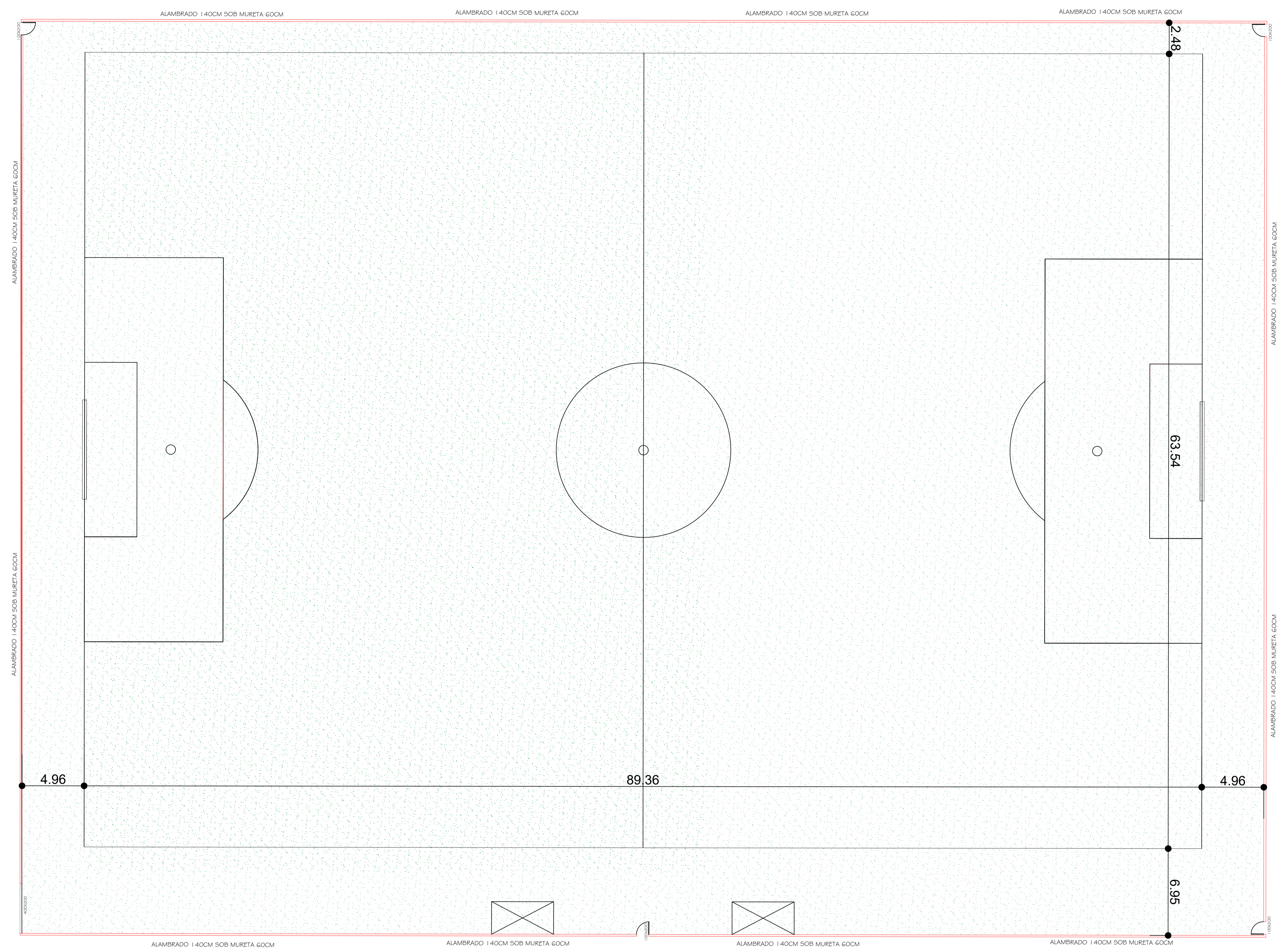
PLANTA BAIXA 1/500
