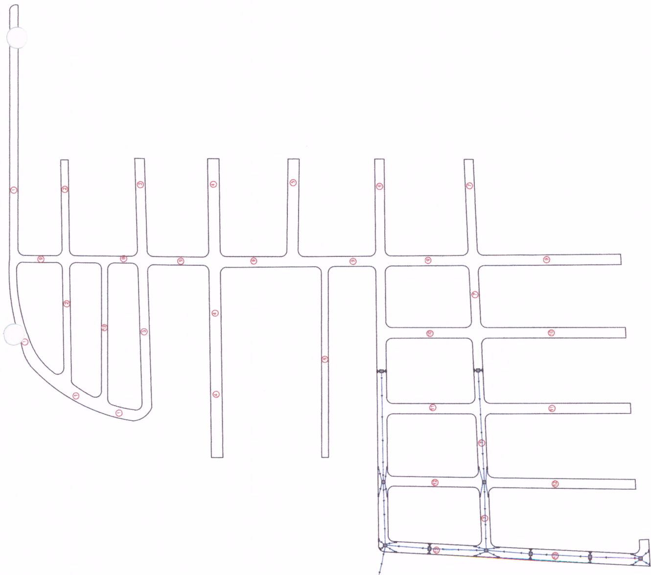
PLANTA BAIXA - DRENAGEM SEM ESCALA
