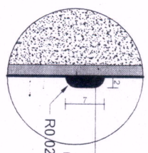
RODA MEIO EM GRANITO BRANCO DALLAS COM ACABAMENTO BOLEADO NAS DUAS EXTREMIDADES
