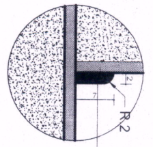
RODAPE EM GRANITO BRANCO DALLAS COM ACABAMENTO BOLEADO
