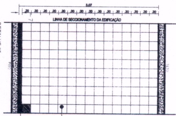
DETALHE 03 PAREDE REVESTIDA ATÉ O TETO
