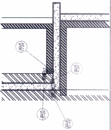
Detalle S3 escala 1:25
