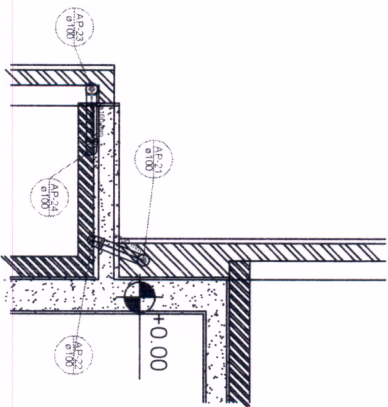
Detalle S6 escala 1:25
