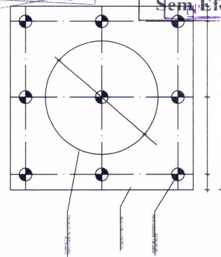
1 LOCALIZAÇÃO DAS ESTACAS
