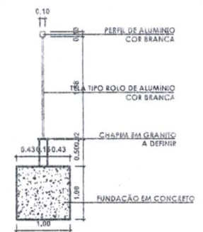
CORTE ESQ. GRADIL
