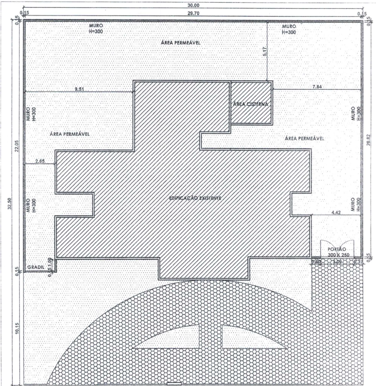
PLANTA BAIXA - MURO USF JUNCADO
